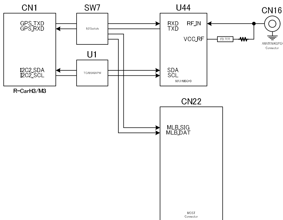
図 4-18 GPS I/F
