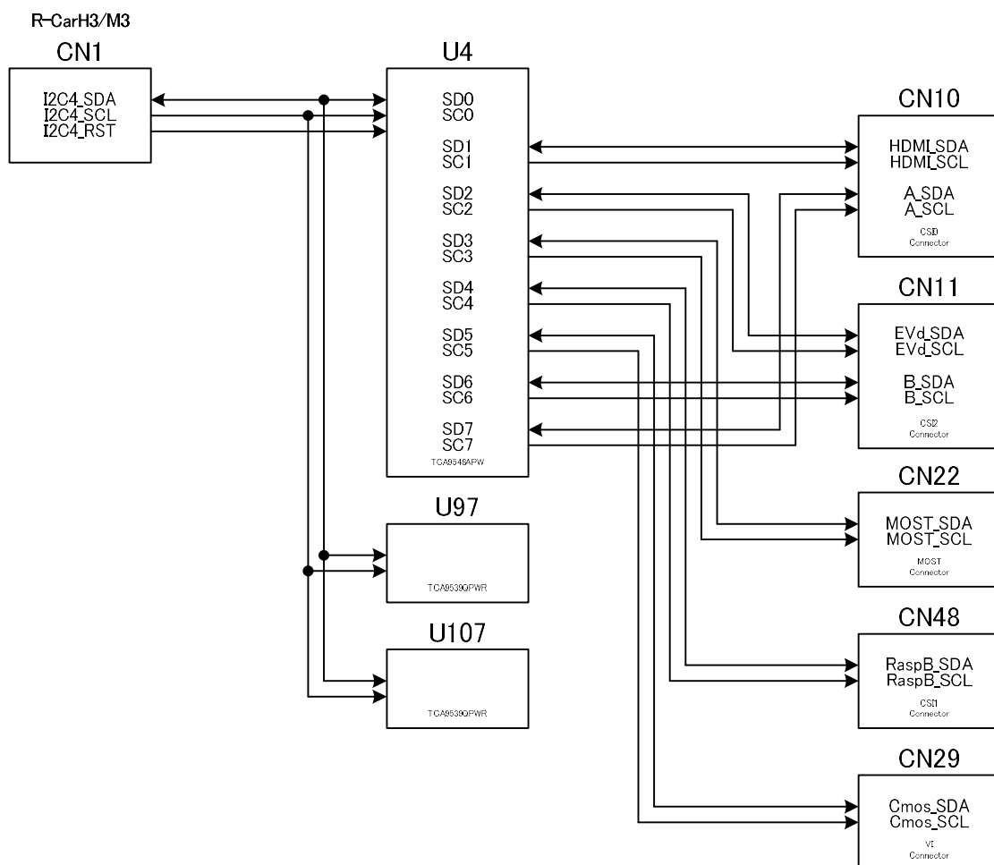
図 4-21b I2C I/F
