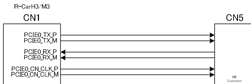
図 4-7 M2 I/F
