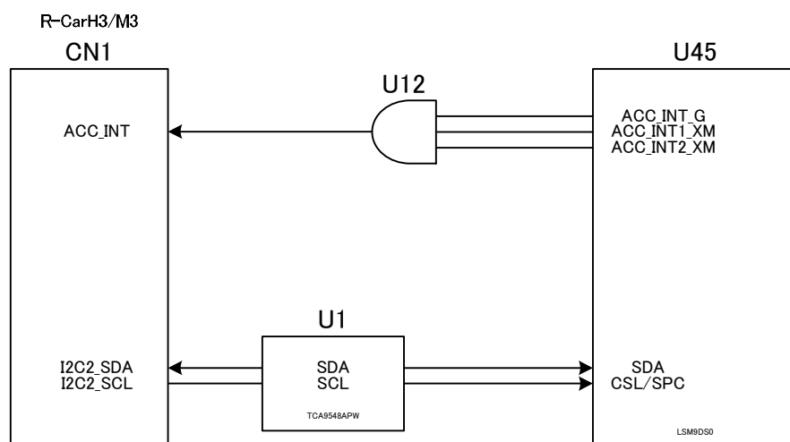
図 4-20 9 軸センサ I/F
