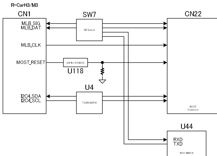
図 4-17 MOST I/F
