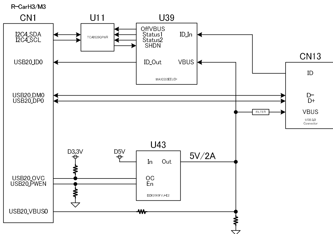
図 4-5 USB 2.0 I/F
