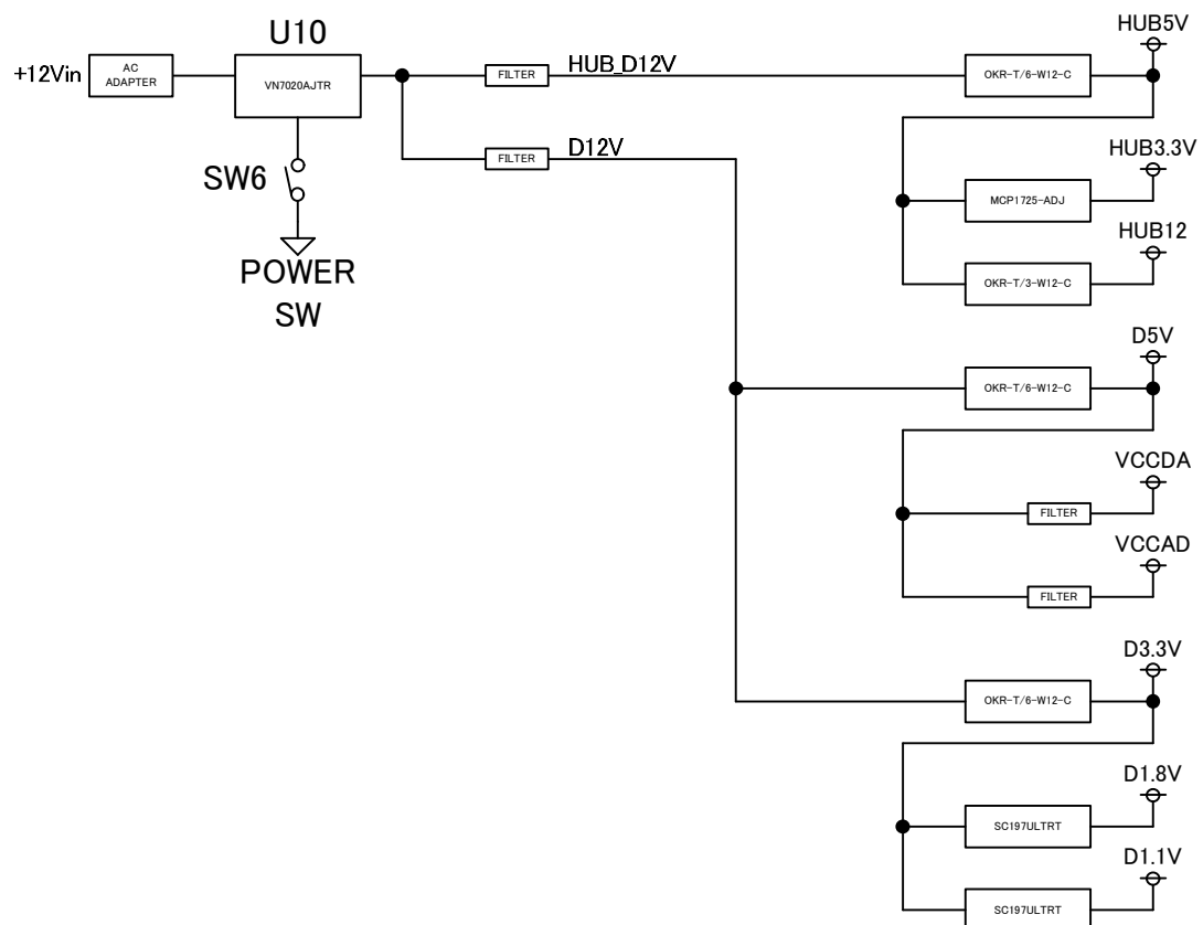
図 4-1 電源系統図
