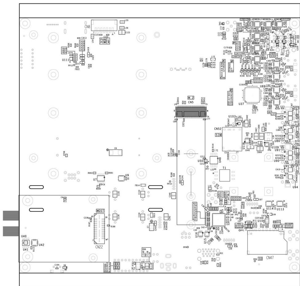
图 9b 基板背面图
