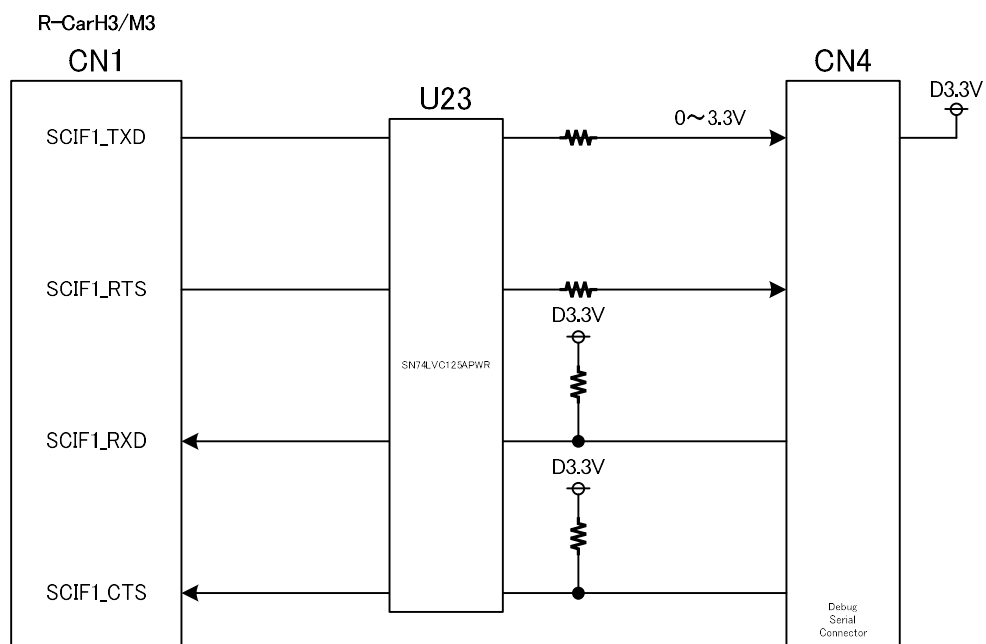
図 4-10 SERIAL I/F
