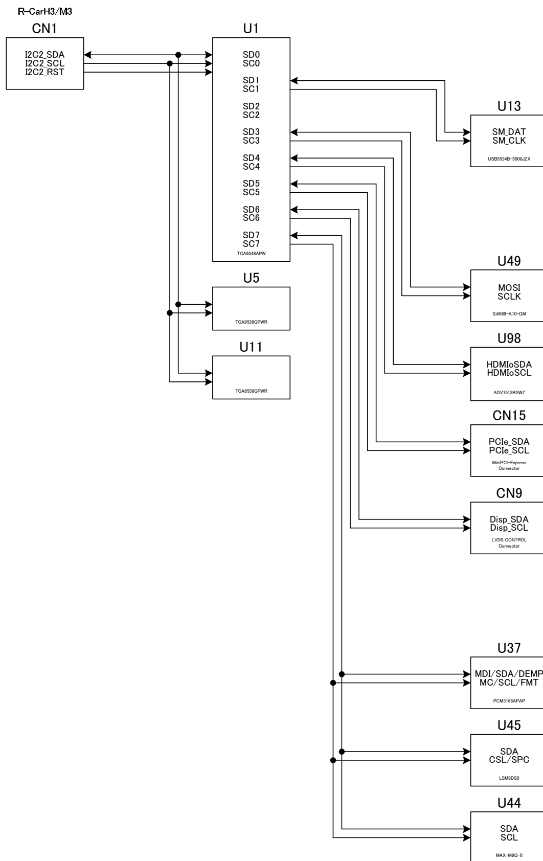
図 4-21a I2C I/F
