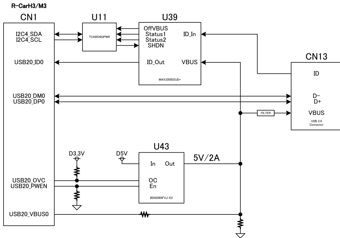
Figure 4-5 : USB 2.0 I/F
